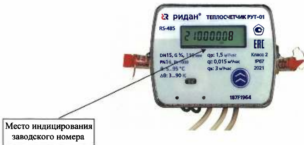
Рисунок 3 – Место индцирования заводского номера
